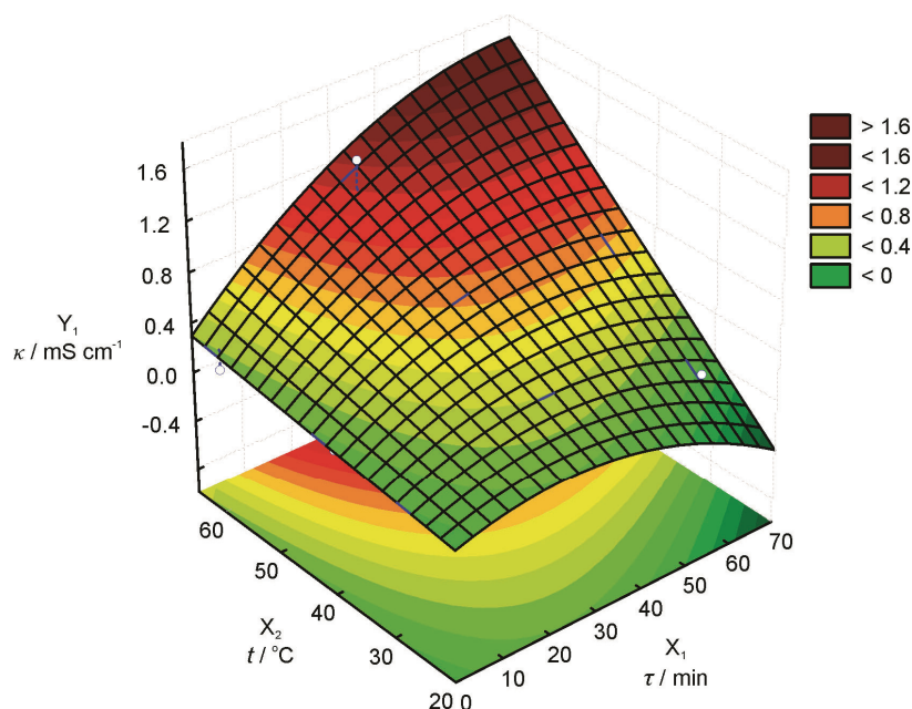
Slika 1. Funkcionalna zavisnost vremena degradacije i temperature na električnu provodljivost kompleksa bakra(II). Figure 1. The functional dependency of degradation time and temperature on the electrical conductivity of copper(II) complex.
